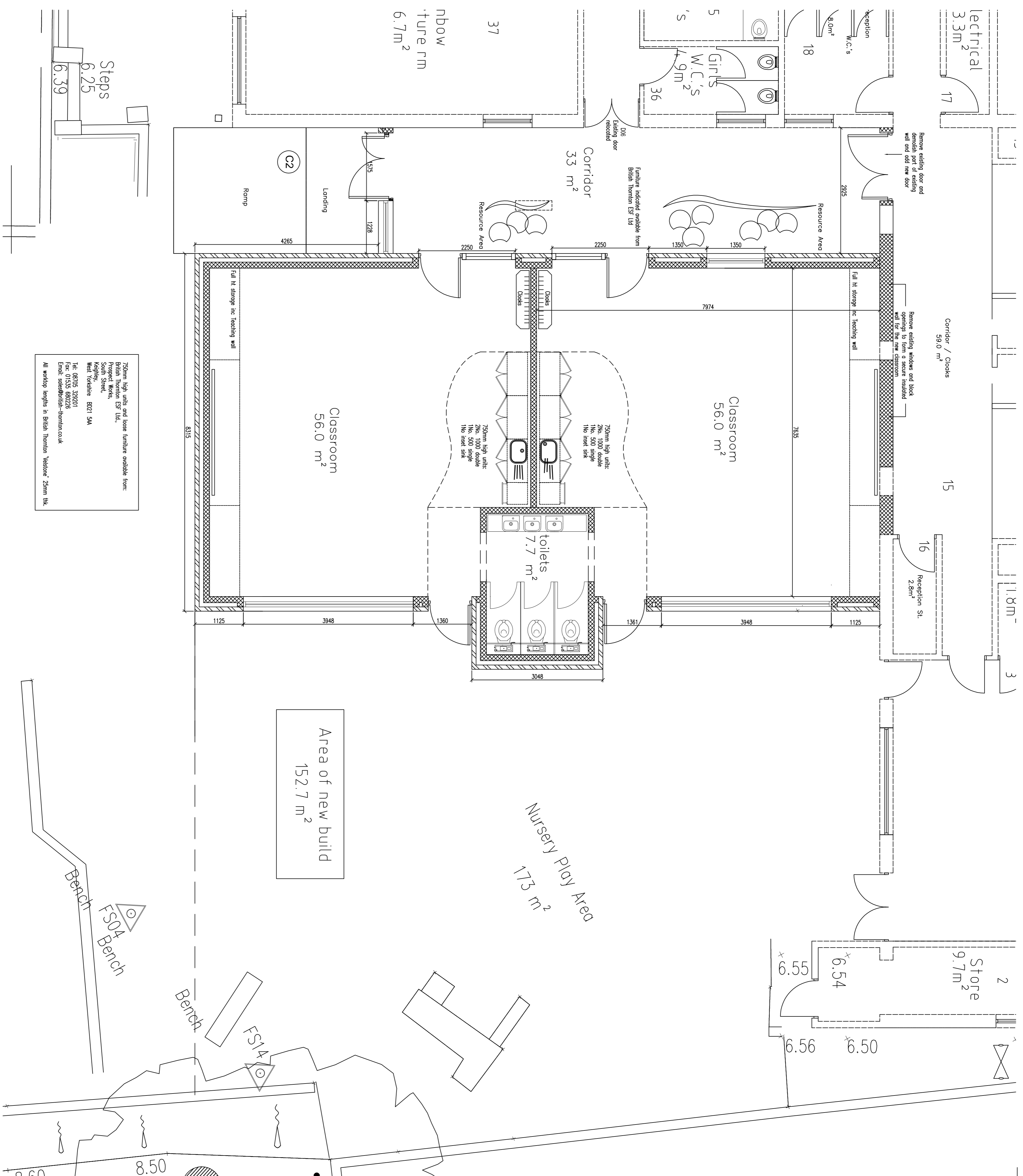
2 Classroom Newbuild Scale: 1:50
